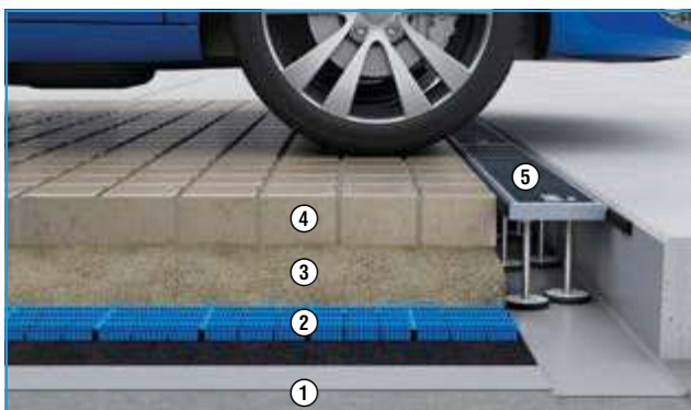
Tunnelartige Entwässerung für befahrbare Betonplatten mit Aqua Drain® HB zur Optimierung der Wasserableitung
