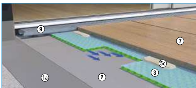
Aqua Drain ® PRO für das punktweise Verlegesystem (s. Technische Datenblatt oder Seite 30)
