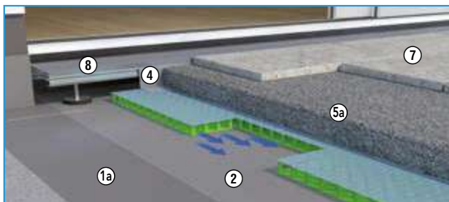
Aqua Drain ® PRO für feste Verlegung (s. Technische Datenblatt oder Seite 16)
