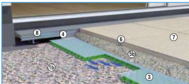
Aqua Drain ® PRO für die lose Verlegung (s. Technisches Datenblatt oder Seite 18)
